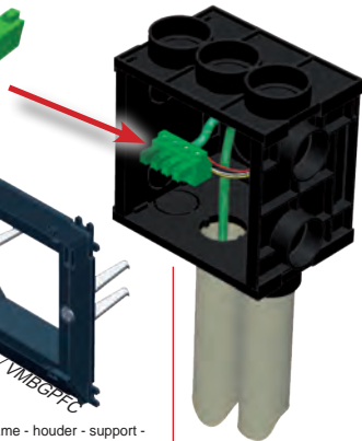
mounting box - inbouwdoos - boîte de montage - Einbaudose - caja de montaje
